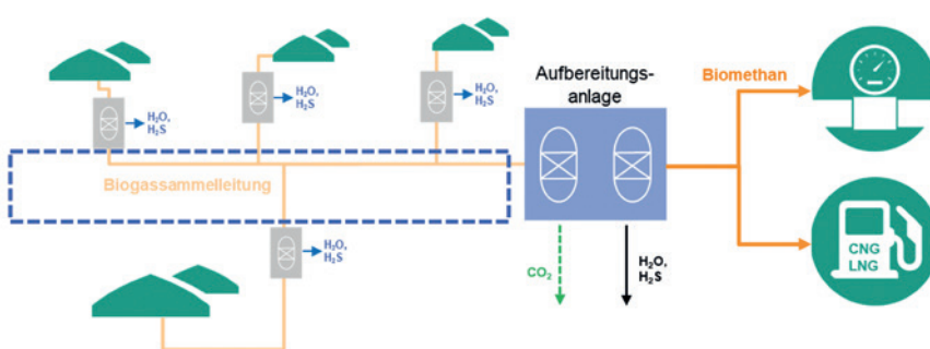
Abb. 5: Sammelleitungen für Biogas
