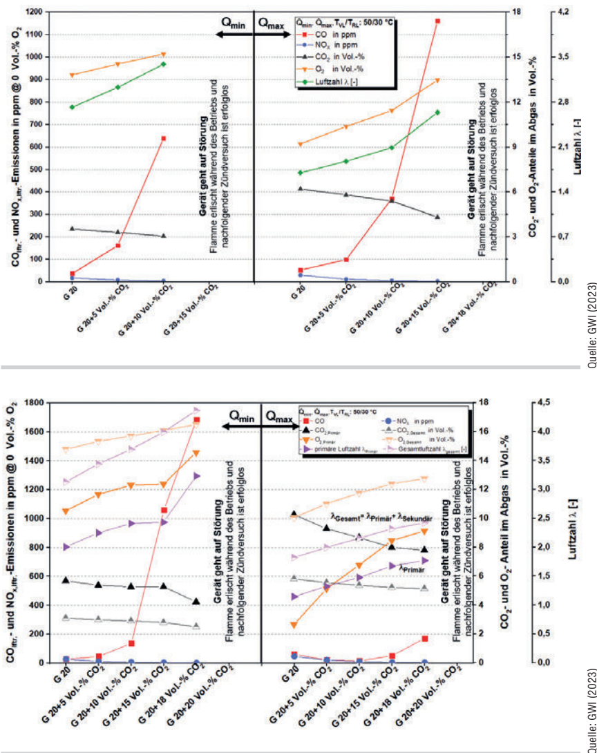
Abb. 2 und 3: Ergebnisse der Laborversuche
